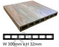
ROFILE Stair se 300 x 32 SC30032
